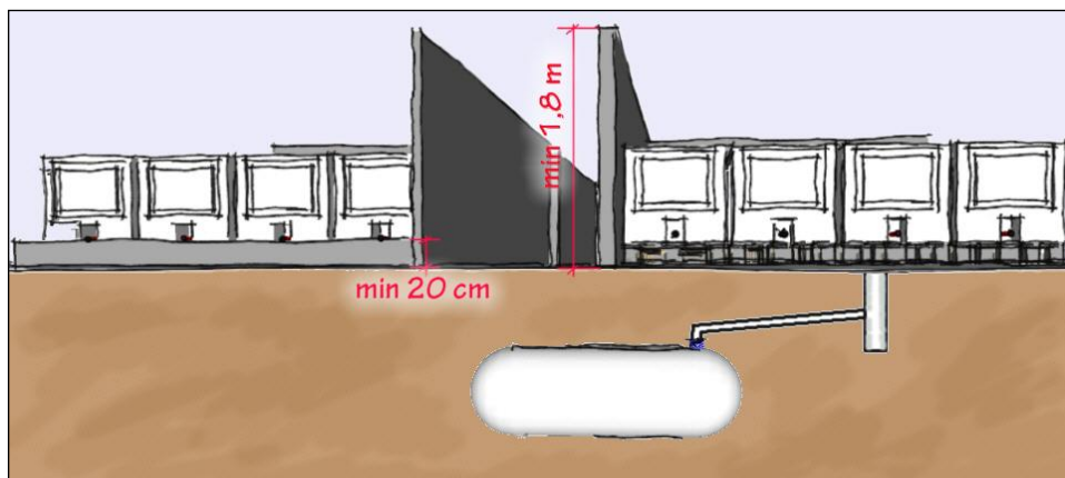
Figur 9: Flammeskærmene bør have en højde på mindst 1,8 m og højst 3 m.
