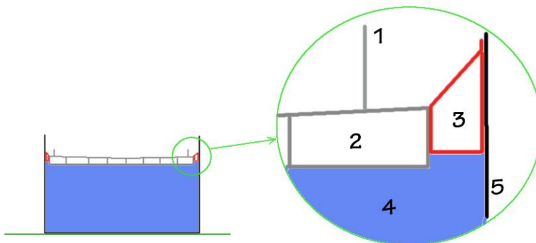
Figur 58: Skitseret detalje af flydetagets forbindelse til tankinderside: 1. Skumbarriere, 2. Hulrum i Double Deck, 3. Rim-seal, 4. Væske, 5. Tanksiden.
