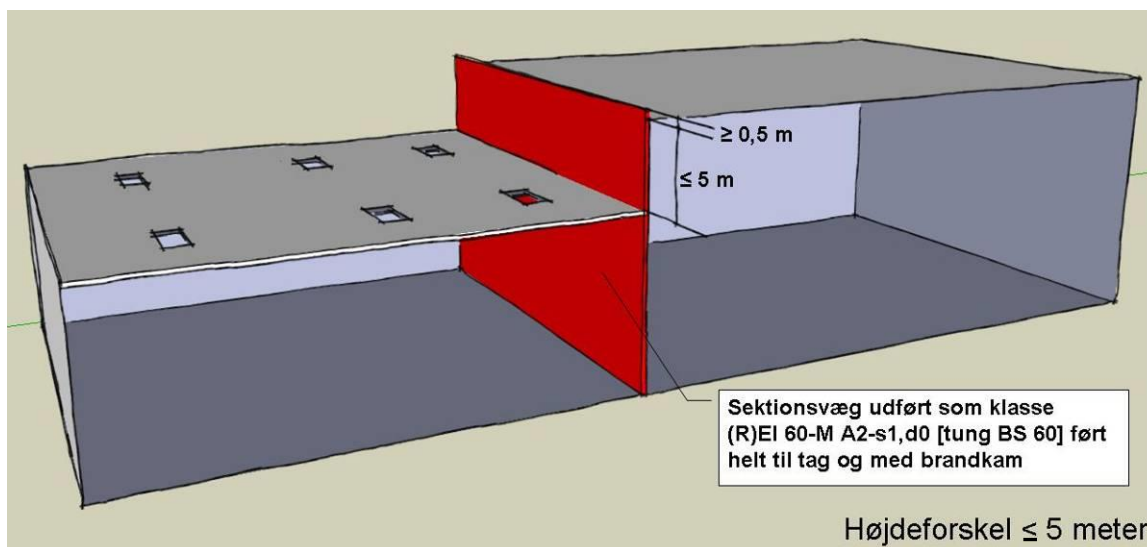
Figur 29: Sikring mod høj-lav brandsmitte, hvor den højere bygnings tag er mindre end eller lig med 5 m over den lavere bygnings tag. Løsning med brandkam.
