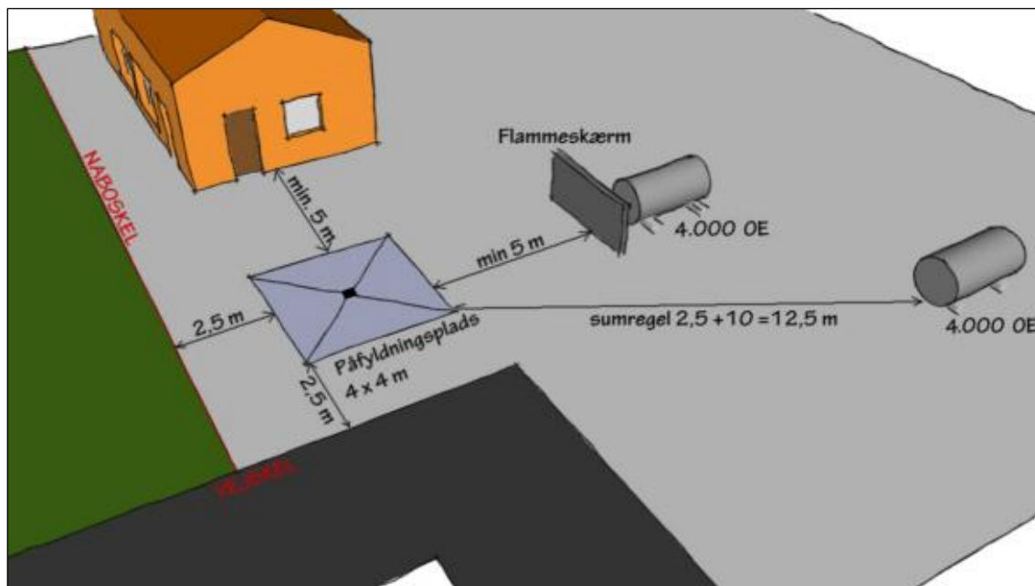
Figur 43: Et eksempel på afstandskrav i forbindelse med en påfyldningsplads. Der må højst være én bygning med mere end 2 etager inden for en afstand af 10 m fra påfyldningspladsen.
