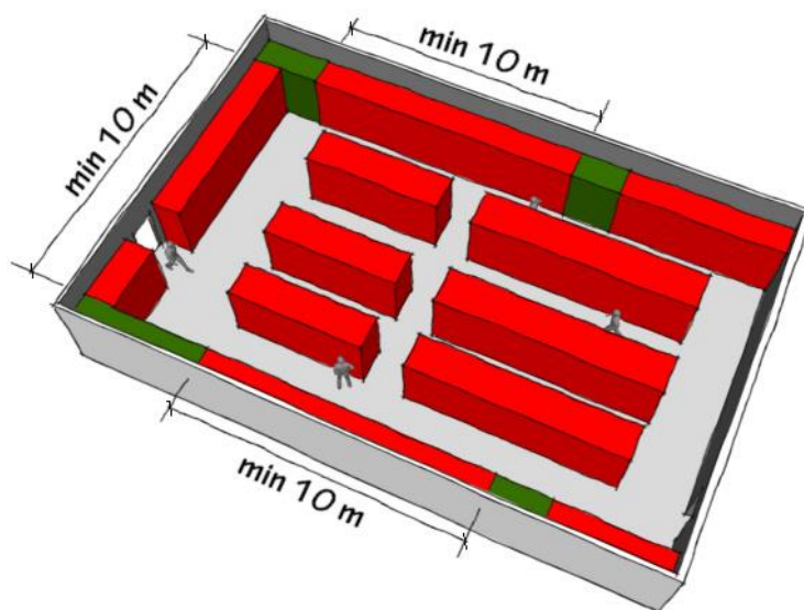
Figur 5: Indbyrdes placering af brandfarlige væsker i butikker uden brug af brandskabe.
