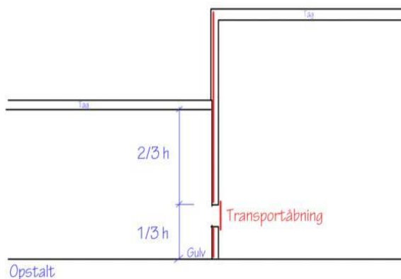
Figur 33: Placering af en transportåbning.
