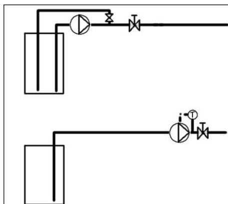
Figur 17: Sikring mod overophedning med omløb (øverst) og med termokontakt (nederst).
