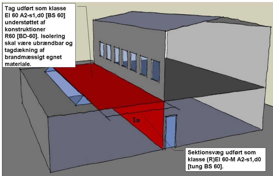
Figur 32: Sikring mod høj-lav brandsmitte, hvor sikringen er udført på den lavere brandsektions tag. Der henvises til vejledningens afsnit om brandkamserstatning for udførelse af tagdækning i brandmæssigt egnet materiale.
