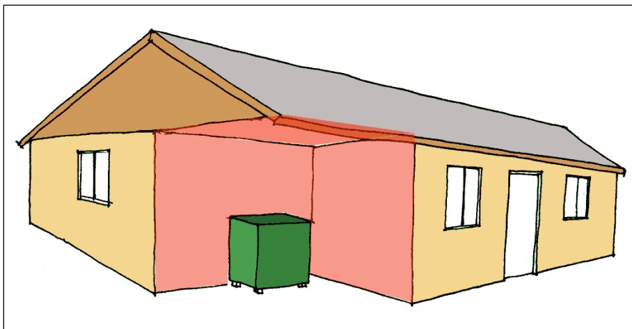
Figur 56: Tank af andet materiale end metal placeret i en carport.
