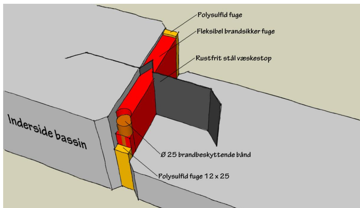
Figur 11: Snit i samling i bassinvæg.
