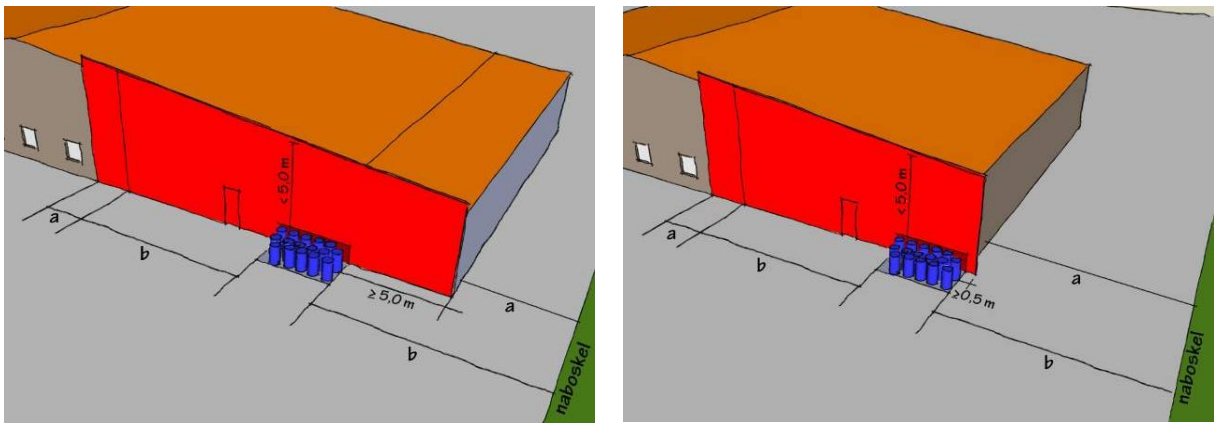
Figur 40: Eksempel på bortfald af den indbyrdes afstand, ved oplag mod bygning, ved etablering af brandsektionsadskillelse inden for den krævede afstand. "Den krævede afstand" svarer til den indbyrdes afstand fundet vha. "sumreglen". I figuren til venstre skal der ikke etableres sikring mod brandsmitte i gavlen, da afstanden overstiger 5 m. I figuren til højre er der vist sikring mod brandsmitte i gavlen, idet brandsektionsadskillelsen er videreført til en afstand af 0,5 m fra bygningens ydervæg. Der er udført en brandkam, idet afstanden fra oplaget til taget er mindre end 5 m.
