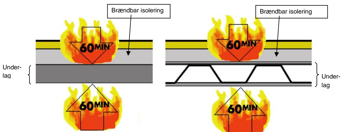
Figur 36: Brændbar isolering i tag på underlag af EI 60 A2-s1,d0.
