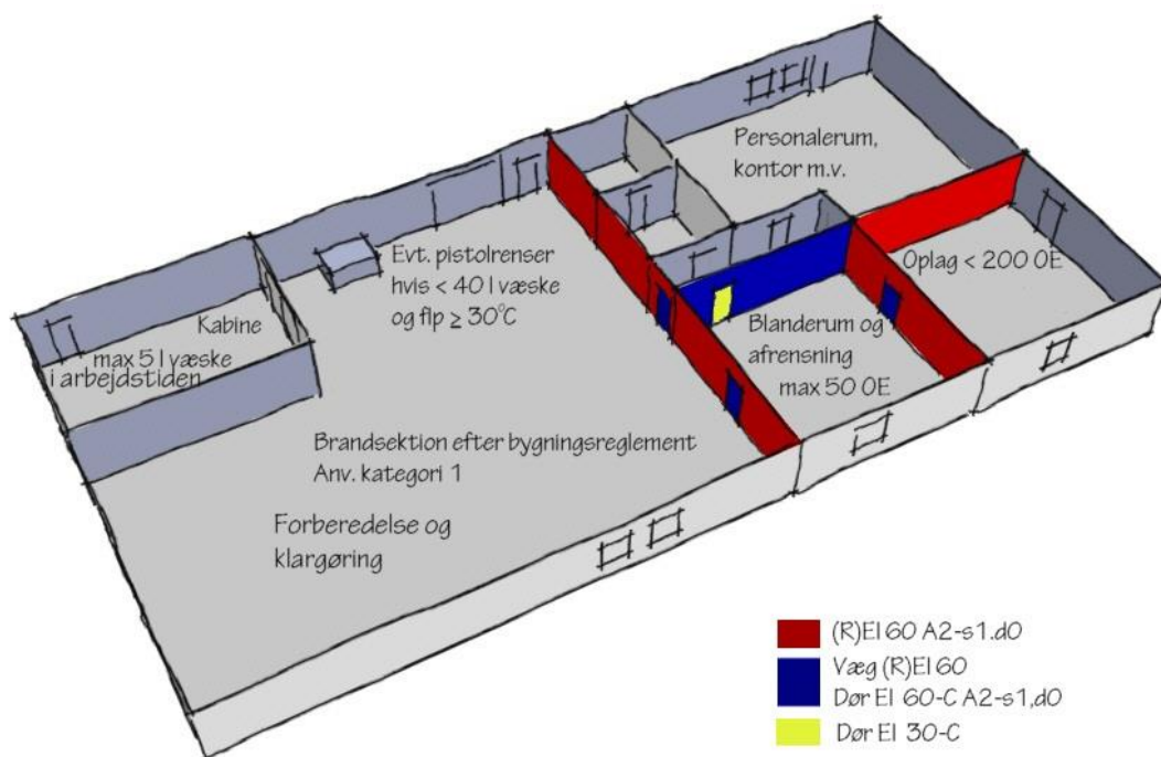
Figur 4: Eksempel på indretning af små autolakererier.
