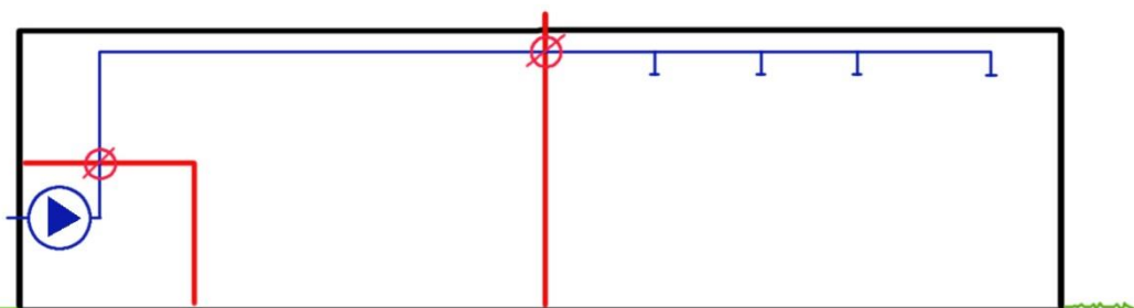
Figur 18: Eksempel på et ventilationsanlæg, der betjener én brandsektion med oplag af kategori A-væsker (må kun betjene én brandsektion). Kanal gennemføringen mellem brandsektionerne og mellem ventilationsrummet og brandsektion er sikret med et brand- og røgspjæld (BRS-spjæld). Kanalerne er udført af mindst materiale klasse A2-s1,d0 af metal med et smeltepunkt på mindst 850 °C.
