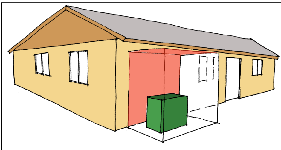
Figur 55: Tank af andet materiale end metal placeret i et skur ved et hus.
