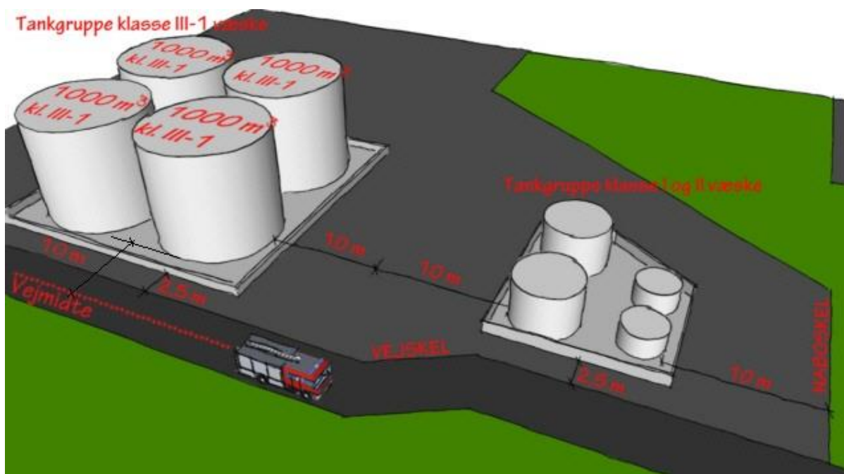
Figur 44: Eksempel på afstande for tanke i grupper til nabo- og vejskel samt indbyrdes afstand.
