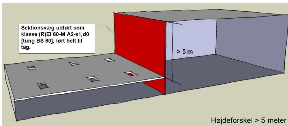
Figur 31: Sikring mod høj-lav brandsmitte, hvor den højere bygnings tag er større end 5 m over den lavere bygnings tag. Ingen krav om brandkam eller brandkamserstatning.
