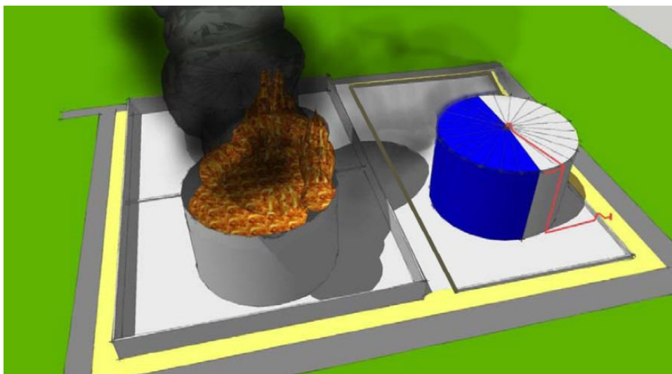
Figur 59: To bassiner, hvor der hhv. er placeret en tank indeholdende klasse III-1-væske og en tank indeholdende klasse I-væske. Det blå felt på tegningen illustrerer kølearealet på tanken med klasse III-1 væske.
