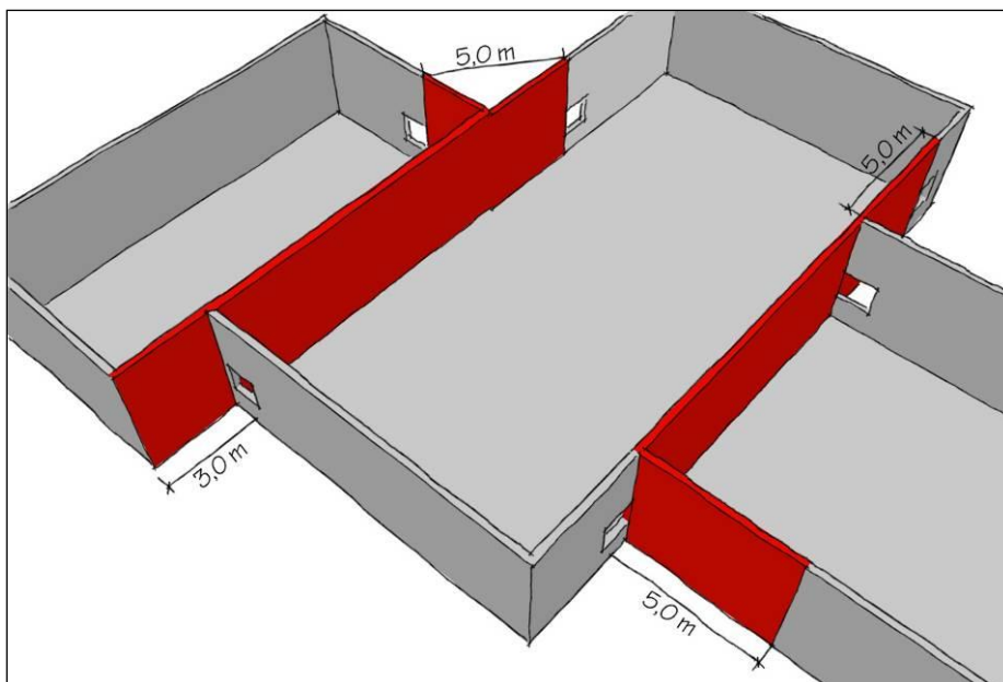
Figur 28: Eksempler på sikring mod vinkelsmitte i ydervægge.
