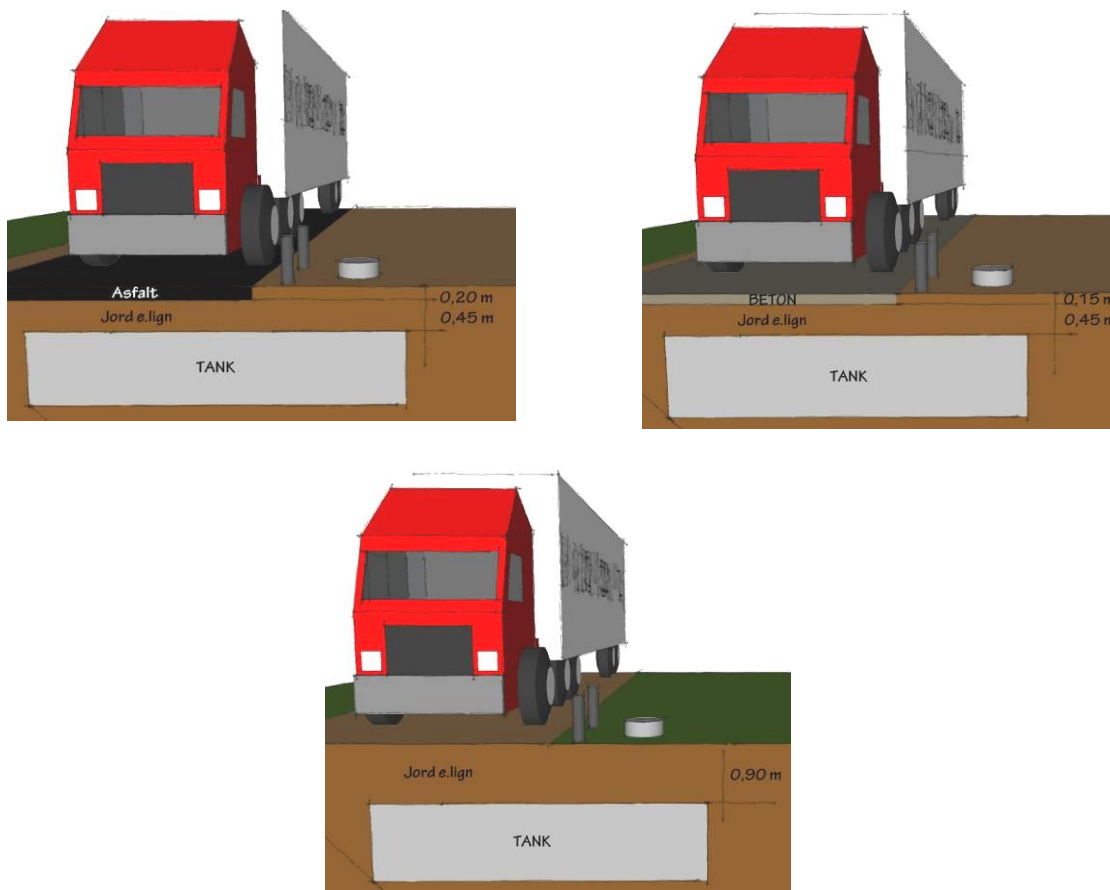
Figur 14: Illustration af forskellige belægninger, herunder tykkelse til beskyttelse af tanken mod trafiklast.
