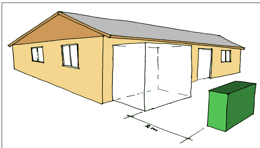
Figur 52: Tank af andet materiale end metal placeret i det fri i en afstand af 2 m fra et skur.
