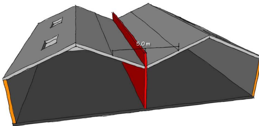
Figur 23: Udførelse af brandkam.
