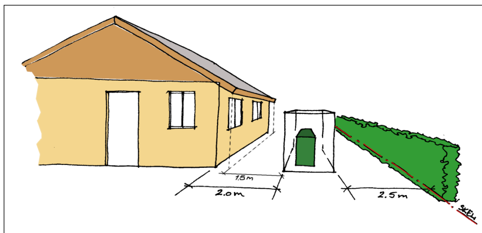
Figur 53: Afstandskrav for en tank af andet materiale end metal placeret i et skur.
