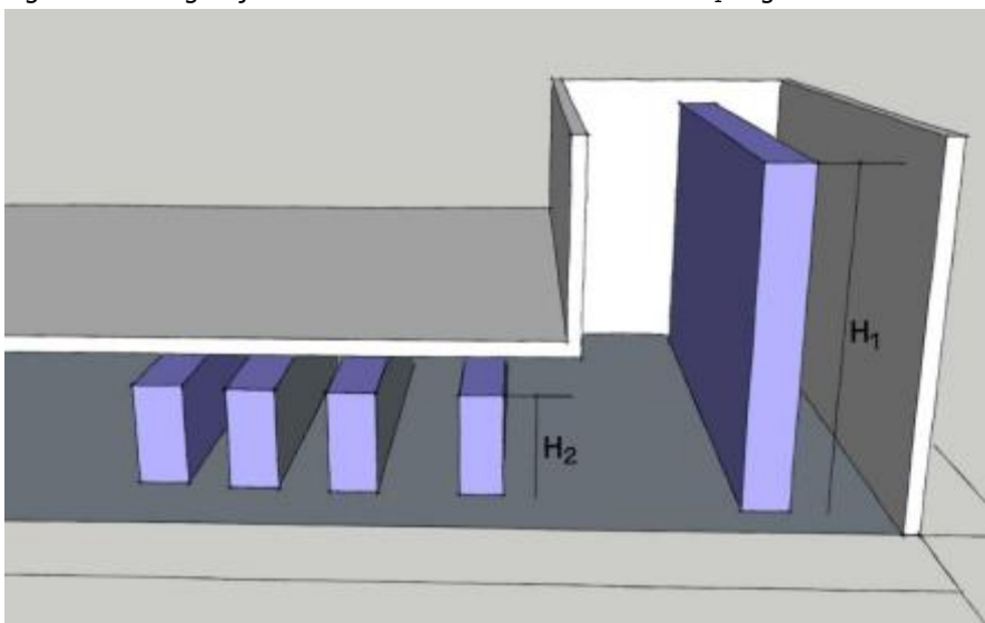
Figur 1: Stablingshøjde i brandsektion med indskudt dæk. H_1 angiver største stablingshøjde, målt fra gulv.
