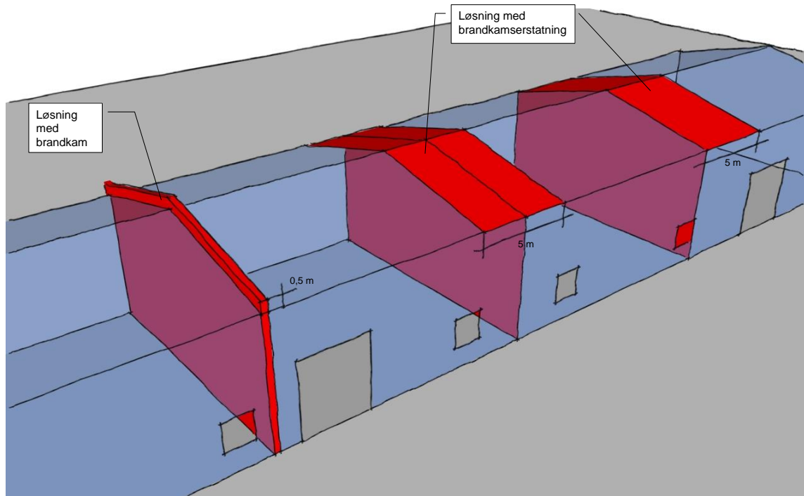
Figur 25: Illustration af løsning med brandkam og brandkammerstatning.
