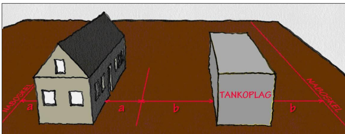
Figur 38: Princip for fastlæggelse af indbyrdes afstandskrav (sumregel).
