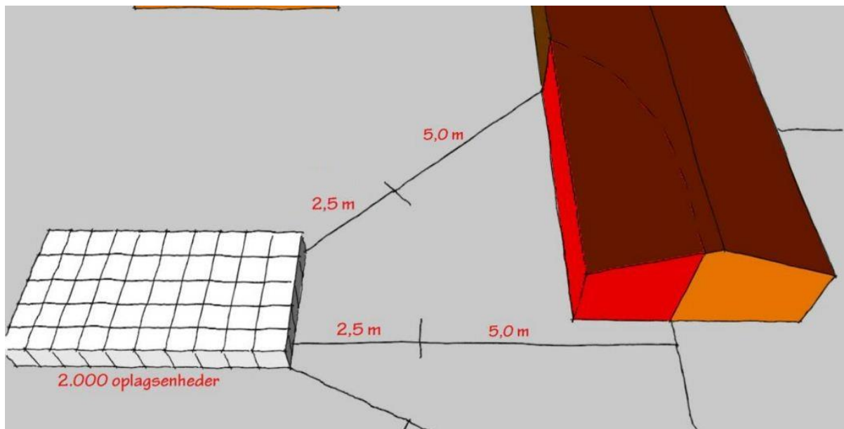
Figur 41: Nedsættelse af den indbyrdes afstand ved oplag mod bygning ved etablering af brandsektionsadskillelse i facaden inden for den krævede afstand (i dette eksempel 7,5 m). Sikring af tag og særlige foranstaltninger mod brandsmitte på gavlvæggen skal kun ske, når den indbyrdes afstand er mindre end 5 m.
