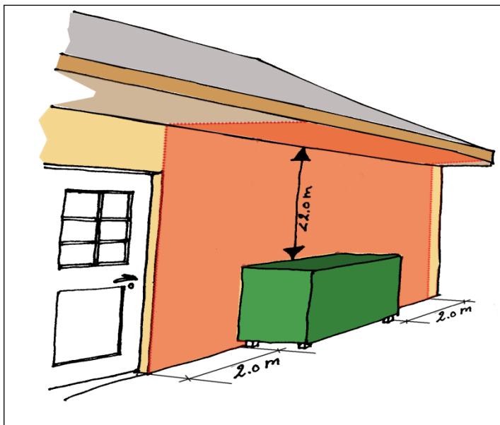
Figur 50: tank af andet materiale end metal placeret i det fri ved et hus.
