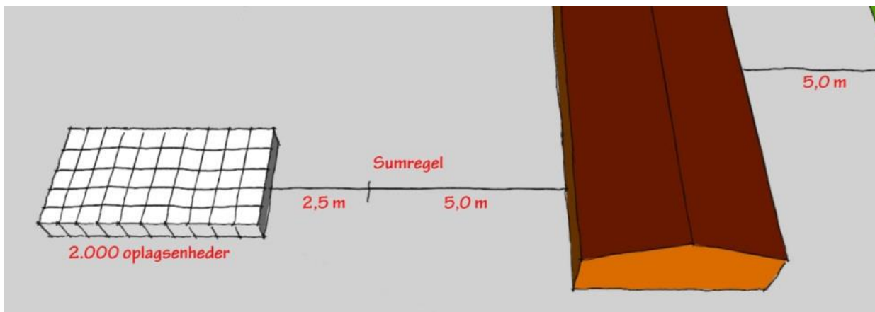
Figur 39: Et eksempel, hvor det indbyrdes afstandskrav er opfyldt.
