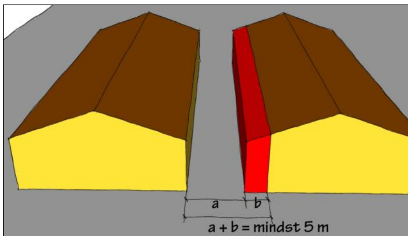
Figur 42: Den krævede indbyrdes afstand er ikke opfyldt mellem to bygninger. Der skal derfor etableres brandsektionsadskillelse, og i en afstand af mindst 5 m skal der i dette eksempel endvidere ske sikring af tag og ydervæg.
