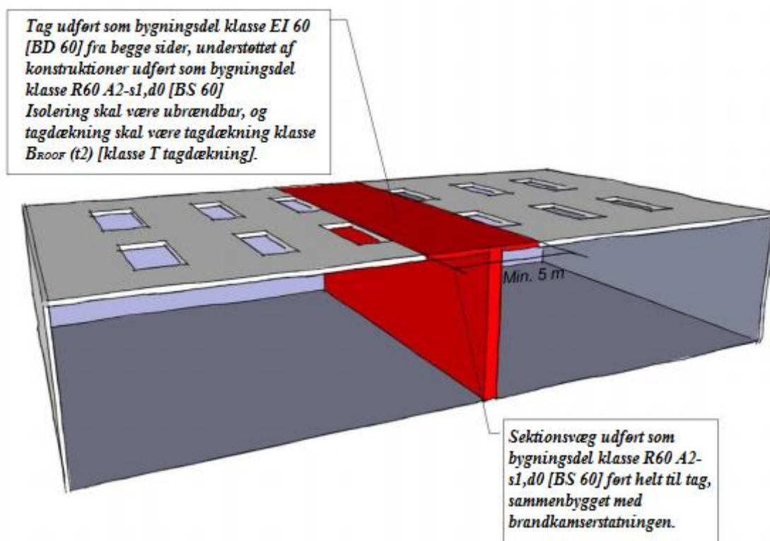
Figur 27: Løsning med 5 m brandkamserstatning med 60 minutters brandmodstandsevne.
