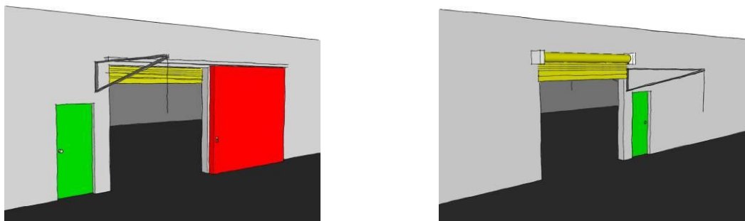
Figur 21: Eksemplet ovenfor viser en løsning med en vandret gående brandskydeport (rød) med lodret hurtiggående uklassificeret port (gul), samt en sidehængt dør, der fungerer som en separat flugtmulighed (grøn). Løsningen bygger på, at den gule lodret gående skydeport holdes lukket. Ved træk i udløser åbnes porten, når der skal trafik gennem, hvorefter den hurtigt lukkes igen. Løsningen er vist fra begge sider af brandsektionsvæggen.
