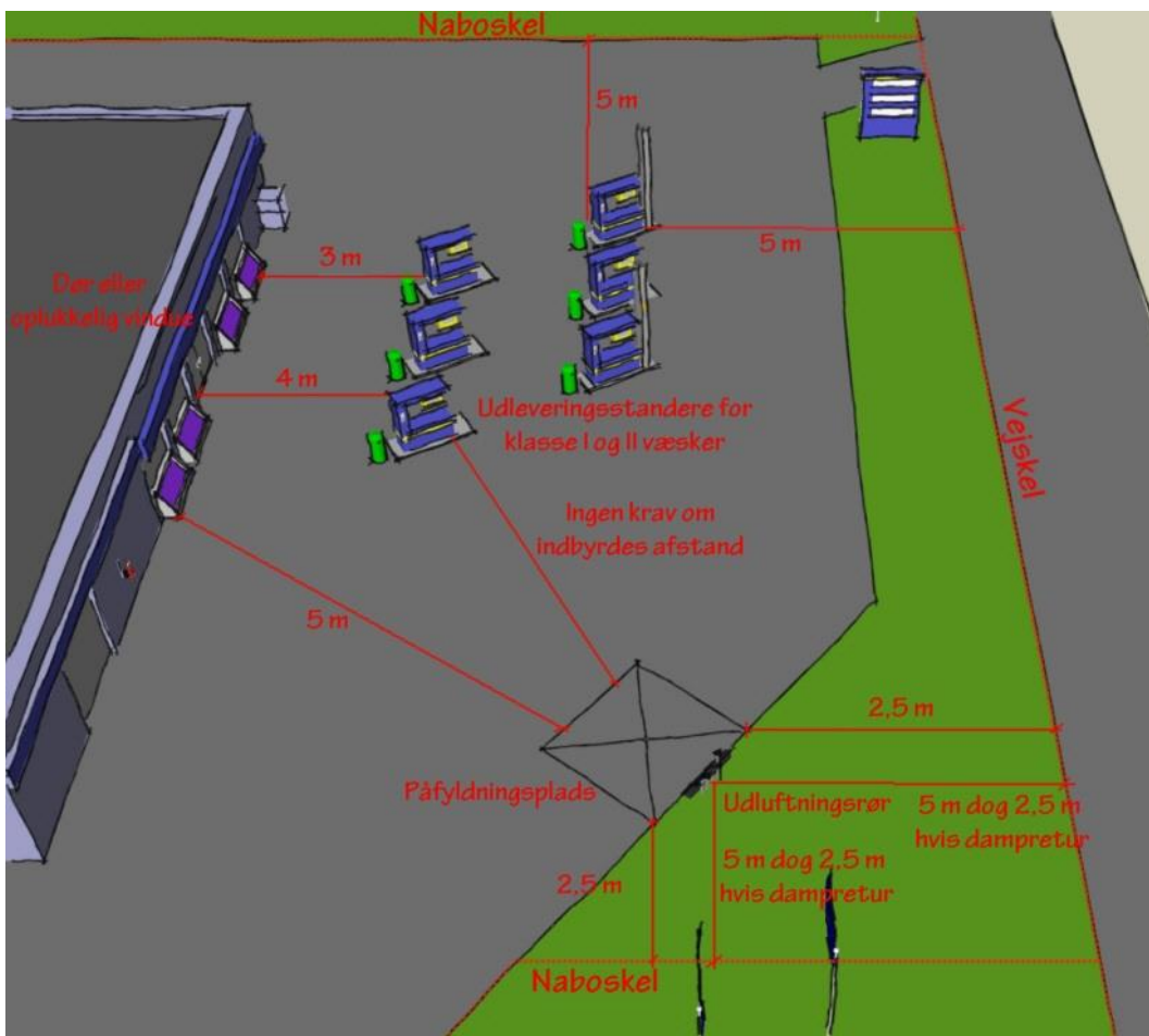
Figur 37: Illustration af afstandskrav, der som minimum skal være opfyldt for salgs- og forbrugtanksanlæg, for væske af klasse I og II.
