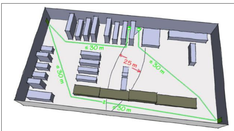
Figur 35: Indretning hvor både 25 og 30 m reglen er opfyldt.
