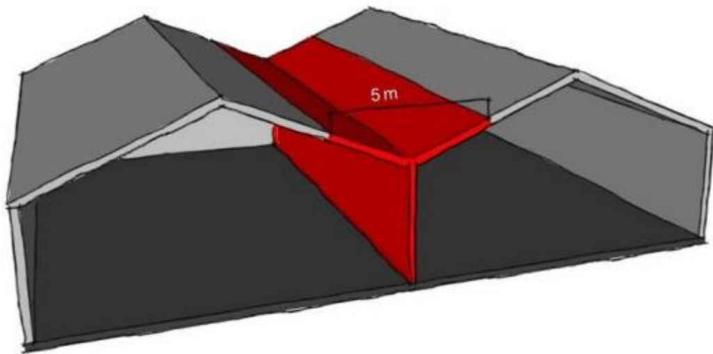
Figur 26: Udførelse af brandkammerstatning med en vandret afstand på 5 m mellem tagfladerne og hvor der er krav til konstruktionen, som understøtter brandkammerstatningen.
