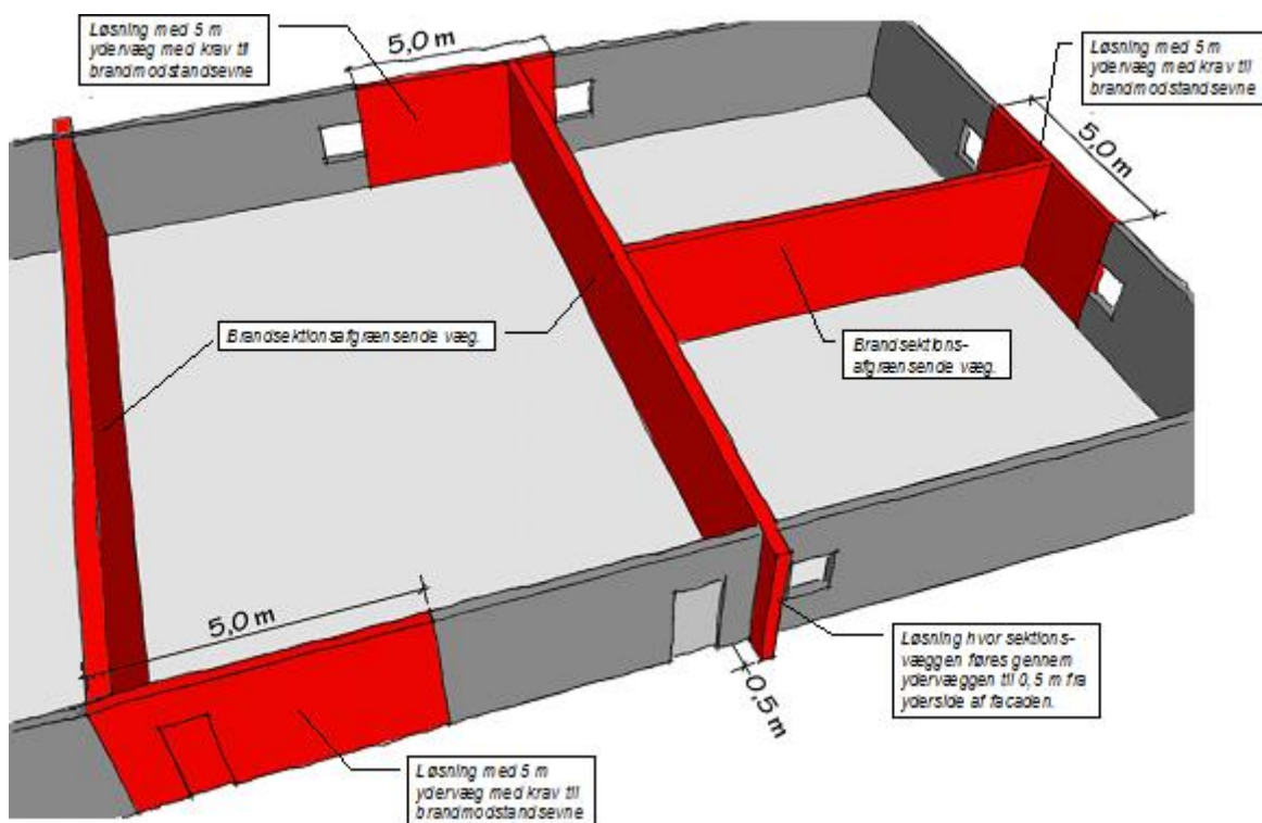
Figur 22: Eksempel på sikring mod brandsmitte (facadesmitte) i ydervæggen.
