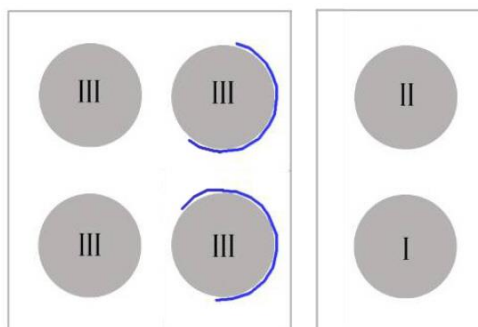
Figur 60: To bassiner med hhv. klasse III tanke og klasse I og II tanke. De to tanke med klasse III væsker, der er i direkte strålingslinje, overrisles hver svarende til \frac{3}{4} tanksvøb (angivet med blå), i tilfælde af brand i tank med enten klasse I eller klasse II væske. Overrisling af tanke kan undlades, såfremt der i forbindelse med skyggevirksomhed ikke kan forekomme farlig varmepåvirkning på tanken.
