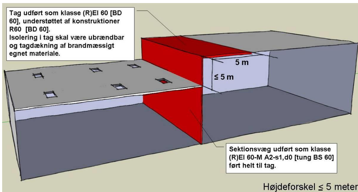
Figur 30: Sikring mod høj-lav brandsmitte, hvor den højere bygnings tag er mindre end eller lig med 5 m over den lavere bygnings tag. Løsning med brandkamserstatning. Der henvises til vejledningens afsnit om brandkamserstatning for udførelse af tagdækning i brandmæssigt egnet materiale.
